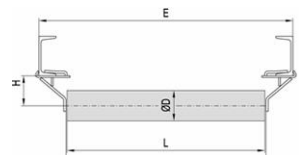
závěsy pro jeden váleček š. pásu 400 - 1400mm
