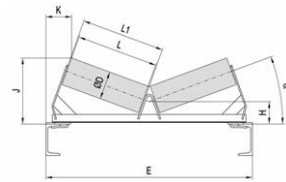
pražec horní dvouválečkový š. pásu 400 - 1000mm
