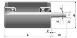
válečky strážní průměr 89 mm průměr 108 mm
