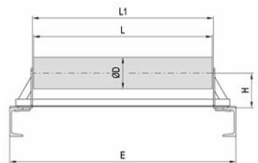
pražec horní jednoválečkový š. pásu 400 - 1500mm
