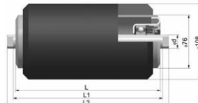
válečky pogumované průměr 108 mm průměr 133 mm
