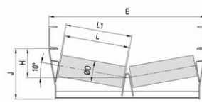
pražec dolní dvouválečkový š. pásu 1000 - 1600mm
