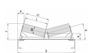
pražec šípovitý dvouválečkový š. pásu 400 - 1000mm
