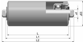
válečky hladké průměr 89 mm průměr 108, 133 mm
