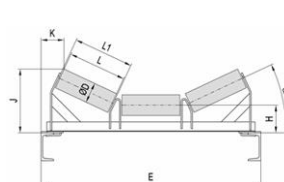
pražec horní tříválečkový š. pásu 400 - 1000mm
