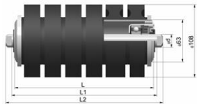
válečky dopadové průměr 108 mm průměr 133 mm
