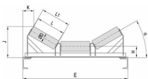
pražec šípovitý tříválečkový š. pásu 400 - 1400mm
