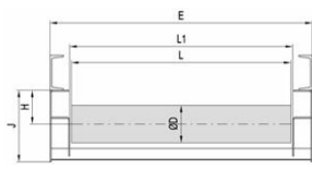
pražec dolní jednoválečkový š. pásu 800 - 1400mm
